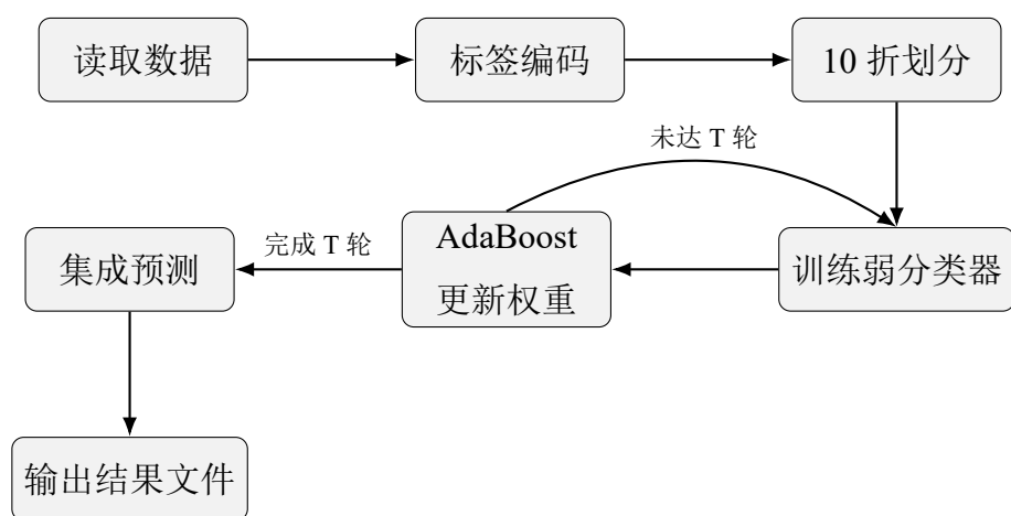
图 1 AdaBoost 实验整体流程图
